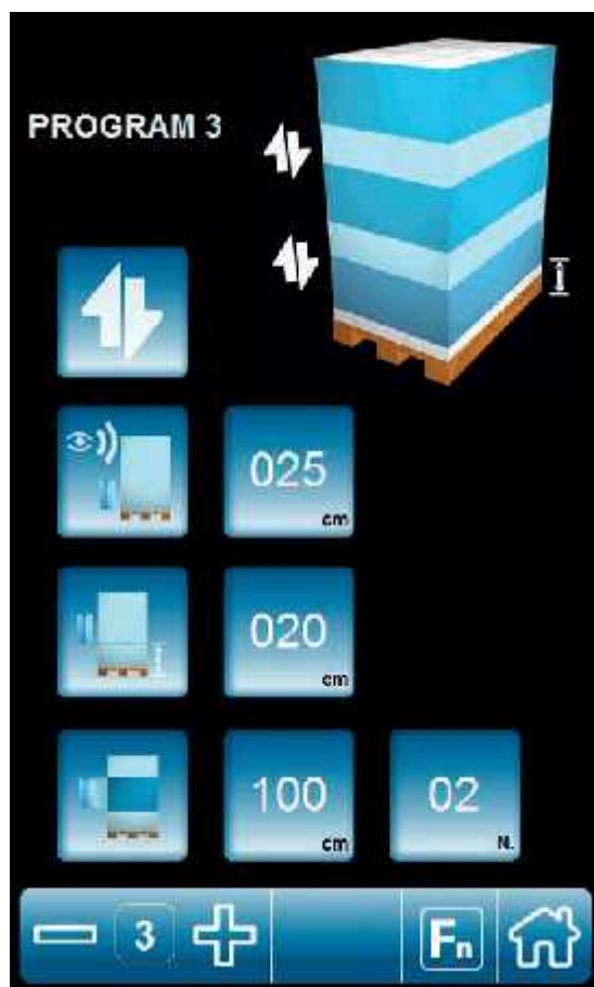
Ciclo mettifoglio Top sheet cycle
